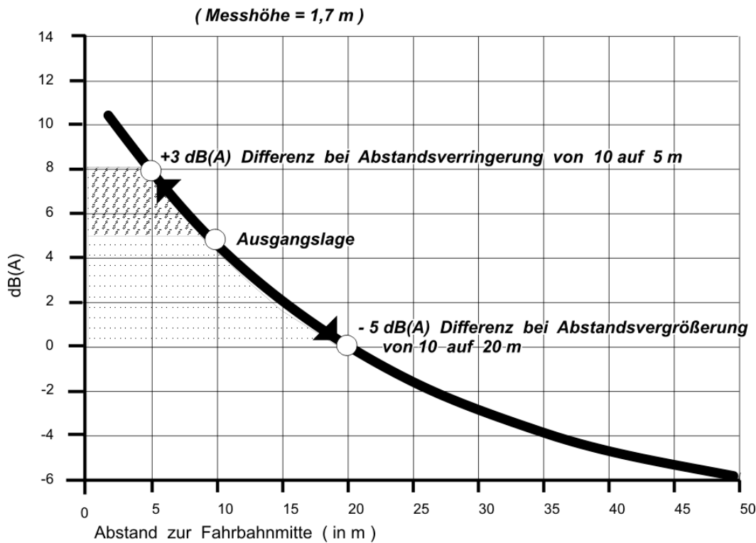
Abbildung 34: Lärmreduzierung durch Erhöhung des Abstands zur Fahrbahnmitte
