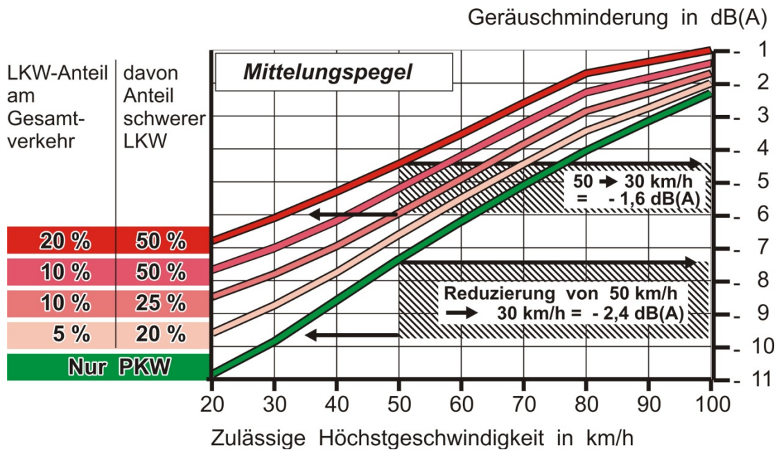
Abbildung 25: Geräuschminderung in Abhängigkeit von Geschwindigkeit und Lkw-Anteil am Gesamtverkehr
