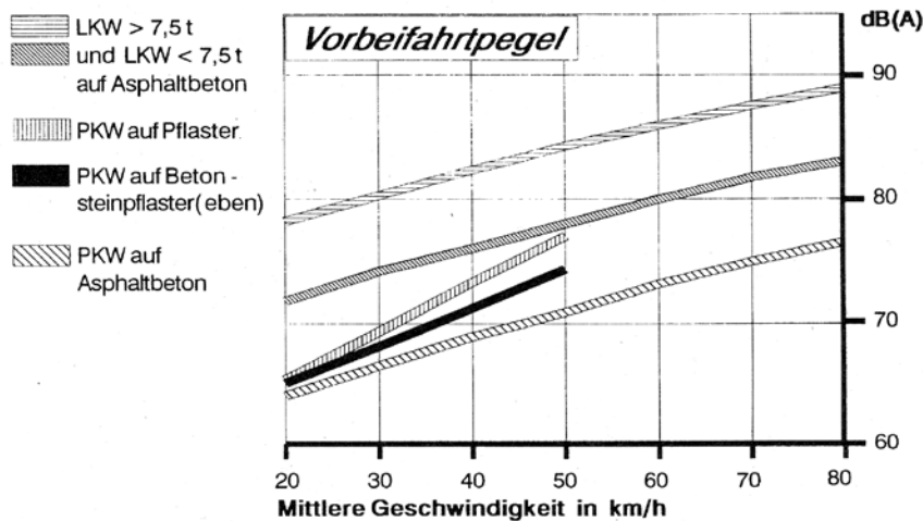
Abbildung 32: Geräuschemissionen (mittlerer max. Vorbeifahrtpegel in 7,5 m Abstand) bei frei fließendem Verkehr
