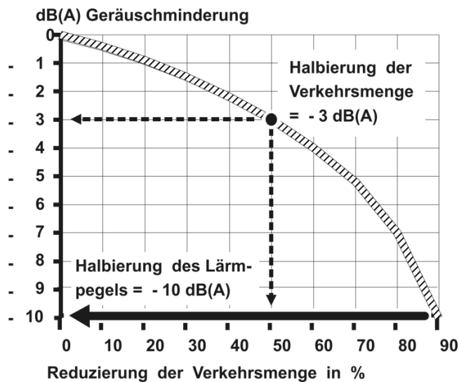
Abbildung 21: Lärminderungspotenzial (Mittelungspegel) durch Reduzierung der Verkehrsmenge
