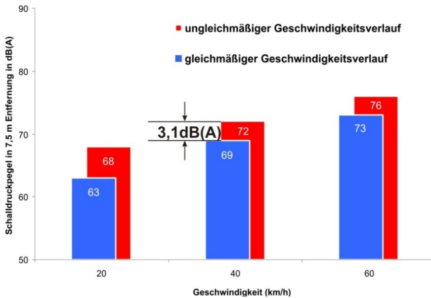
Abbildung 28: Lärminderungspotenzial durch Verstetigung der Geschwindigkeit
