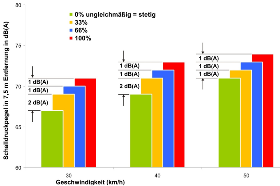
Abbildung 30: Lärminderungspotenzial durch Reduzierung und Verstetigung der Geschwindigkeit
