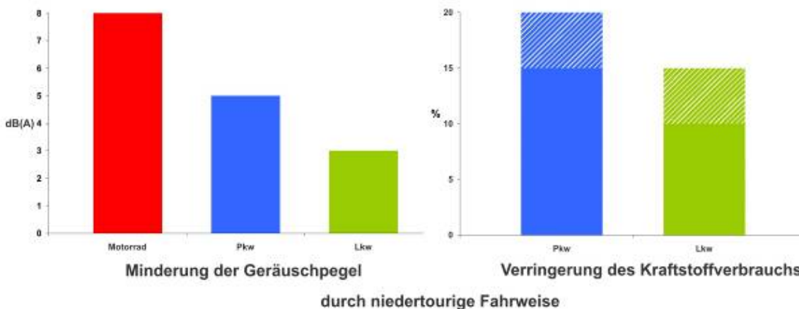
Abbildung 29: Lärminderungspotenzial durch niedertourige Fahrweise
