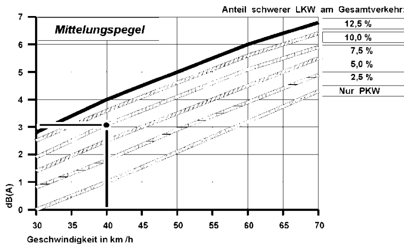
Abbildung 26: Geräuschentwicklung bei ungestörtem Verkehrsfluss (Bezugsbasis: ungestörter Verkehrsfluss, v = 30 km/h, Anteil schwerer Lkw = 0 %)
