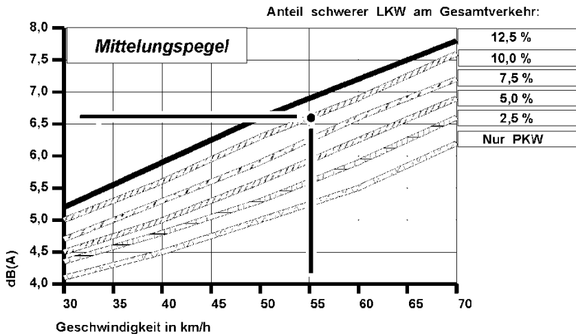
Abbildung 27: Geräuscentwicklung bei gestörtem Verkehrsfluss (Bezugsbasis: ungestörter Verkehrsfluss, v = 30 \text{ km/h} , Anteil schwerer Lkw = 0 %)
